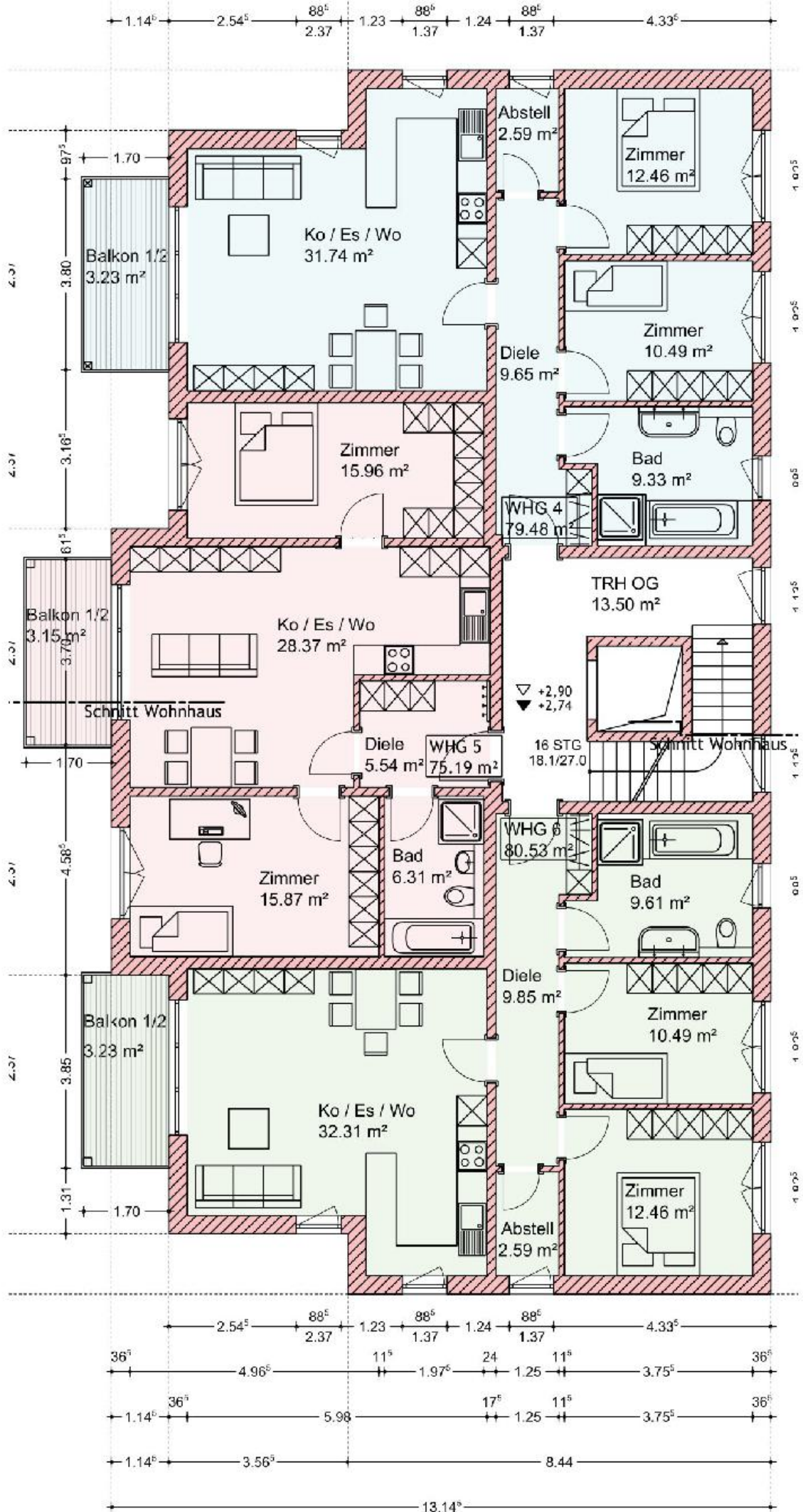
Grundriss OBERGESCHOSS
