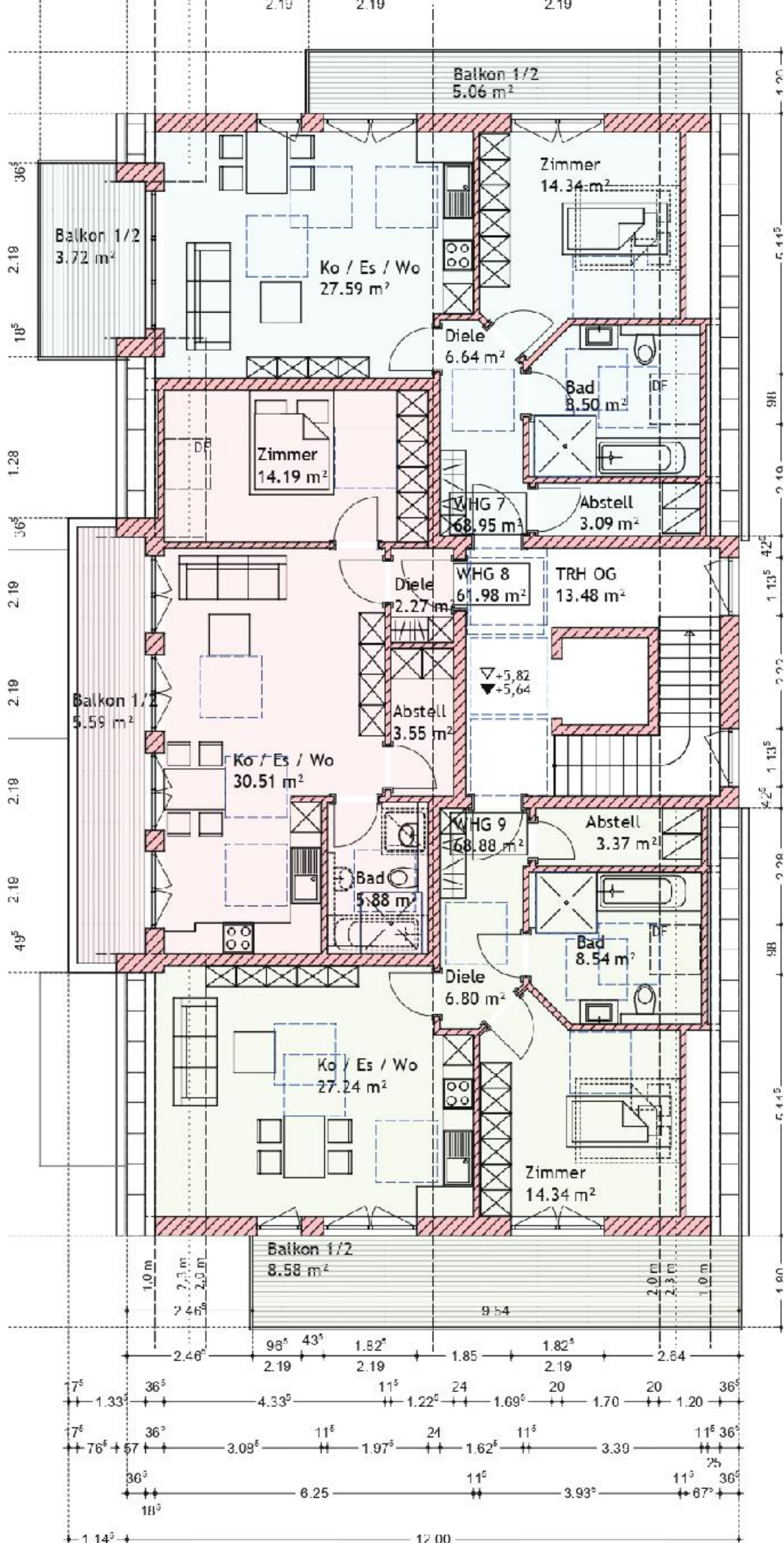
Grundriss DACHGESCHOSS
